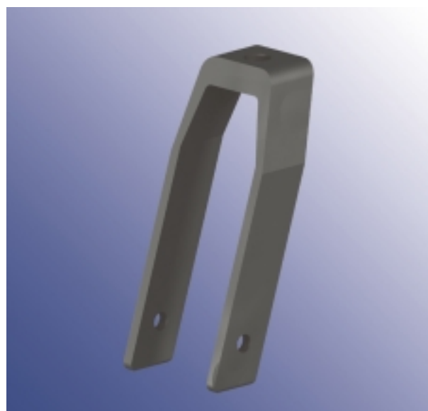
LG-A-150-12S Kiinnitys reikä | Bore hole 12 mm LG-A-150-16S Kiinnitys reikä | Bore hole 16 mm
