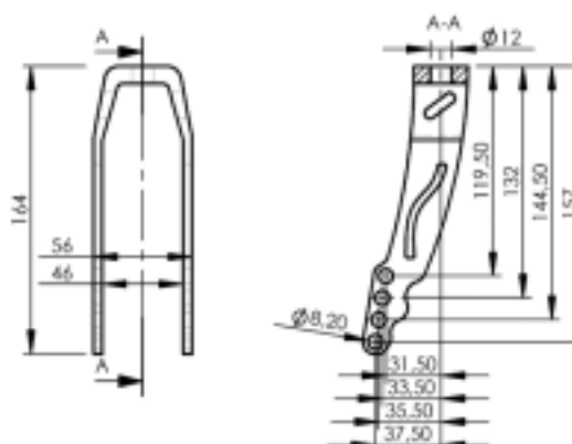
Super light LG-A-SL-200-12S* Kiinnitys reikä | Bore hole 12 mm Super light LG-A-SL-200-16S* Kiinnitys reikä | Bore hole 16 mm
