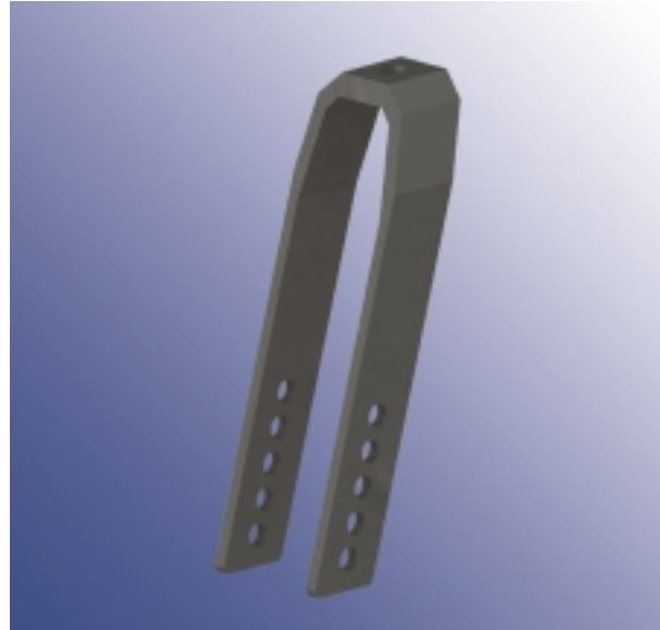
LG-A-200-39-12S Kiinnitys reikä | Bore hole 12 mm LG-A-200-39-16S Kiinnitys reikä | Bore hole 16 mm
